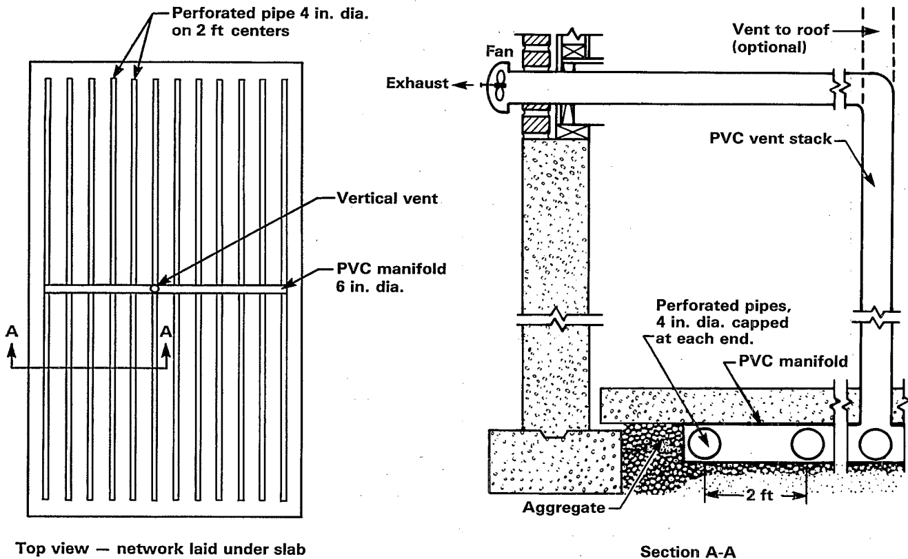
Section A-A
